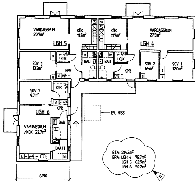
PLAN: ÖVANVÅNING 1:100 (PLANLÖSNING BASUTFÖRANDE 2)
