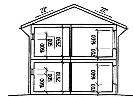
TYPSEKTION 1:100
