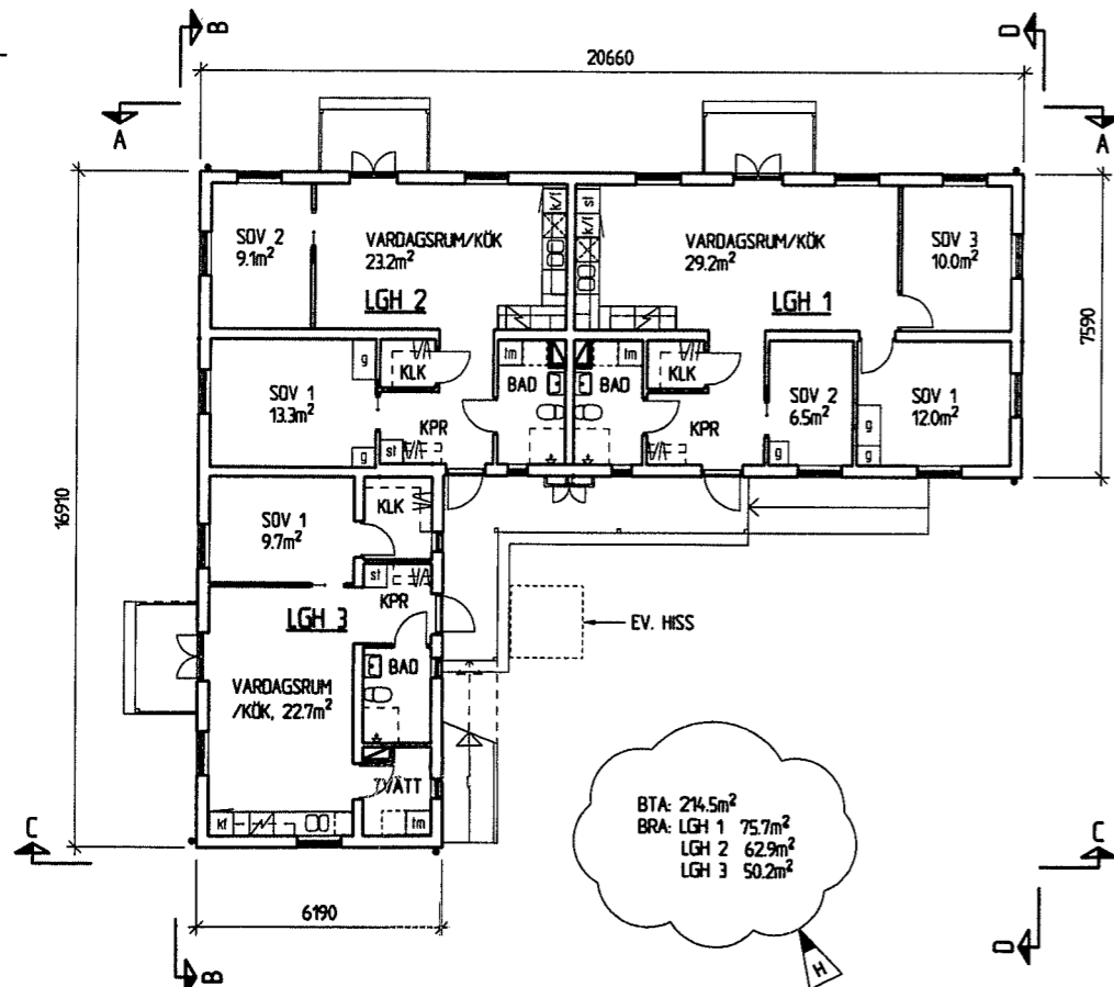
PLAN: BOTTENVÅNING 1:100 (PLANLÖSNING BASUTFÖRANDE 1)
