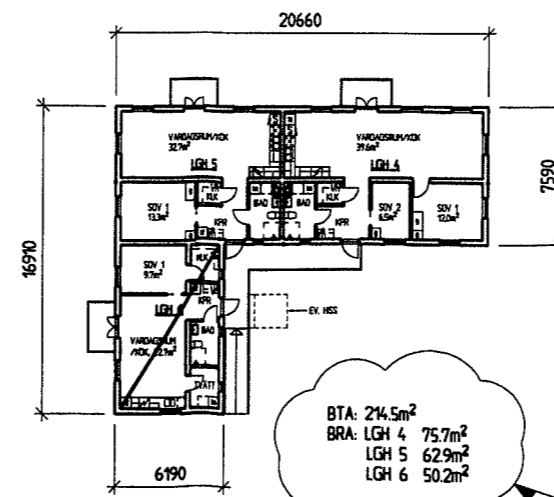
PLAN: PLANLÖSNINGALTERNATIV 1:200 (BASUTFÖRANDE 3)
