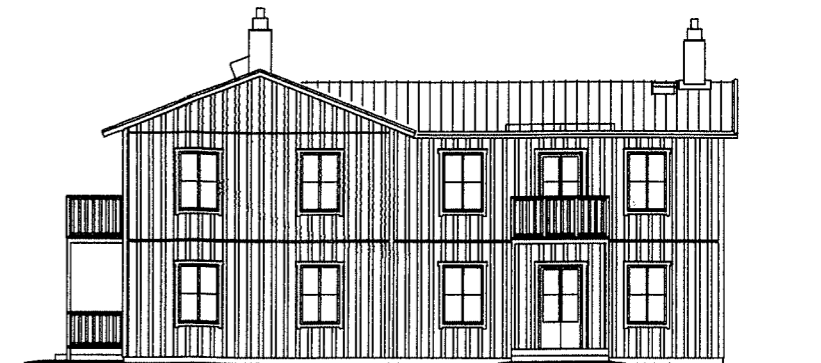
FASAD B-B 1:100
