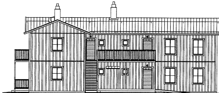
FASAD C-C 1:100
