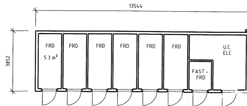
PLAN FÖRRÅDSBYGGNAD TYP 6+UC (TIDIGARE TYP B)
