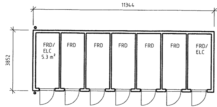
PLAN FÖRRÅDSBYGGNAD TYP 6+1 (TIDIGARE TYP A)
