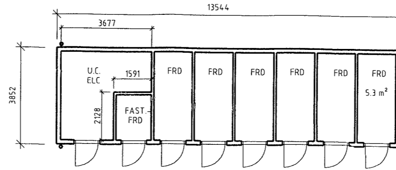
PLAN FÖRRÅDSBYGGNAD TYP 6+UCS (TIDIGARE TYP C)
